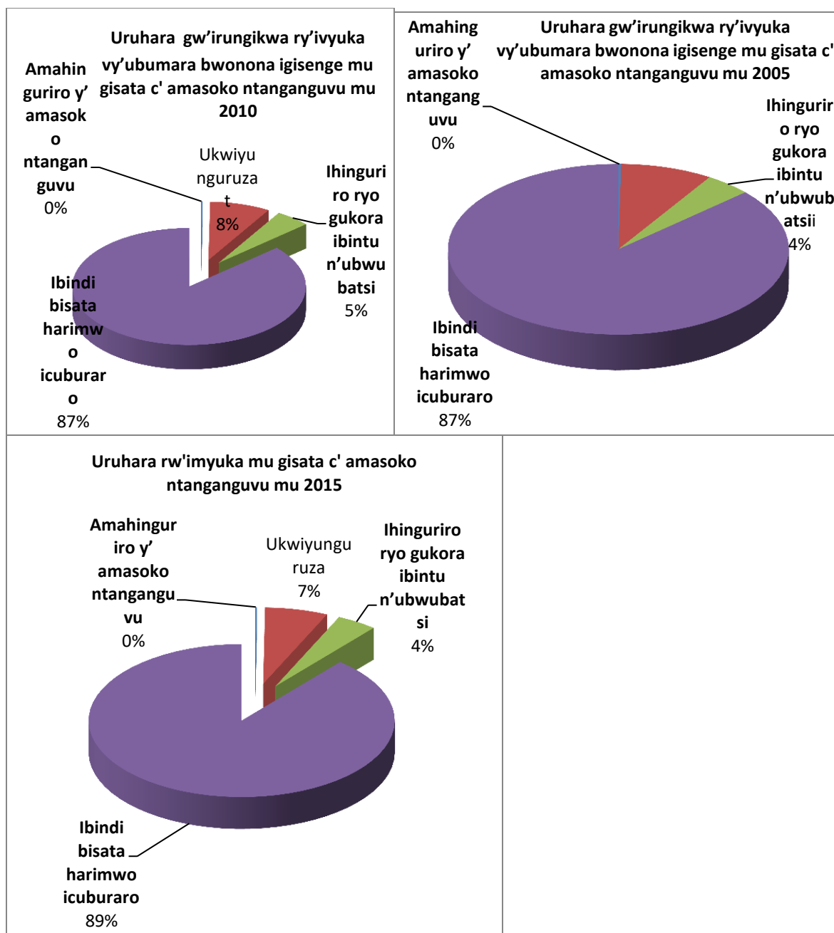
Igicapo ca 9 : Uruhara gw'irungikwa ku gisata c'amasoko ntanganguvu
