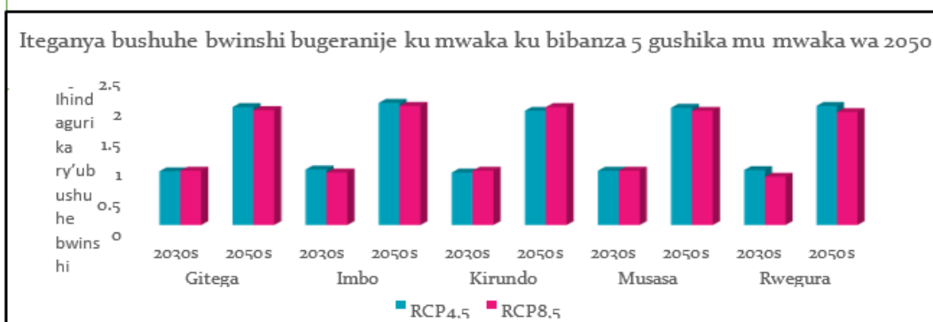
Iyongerekana ry'ubushuhe buke bushoboka gushika mu mwaka wa 2030 na 2050 ku bibanza vy'ibipimo ndangagihe vya Gitega, Kirundo ; Musasa na Rwegura
