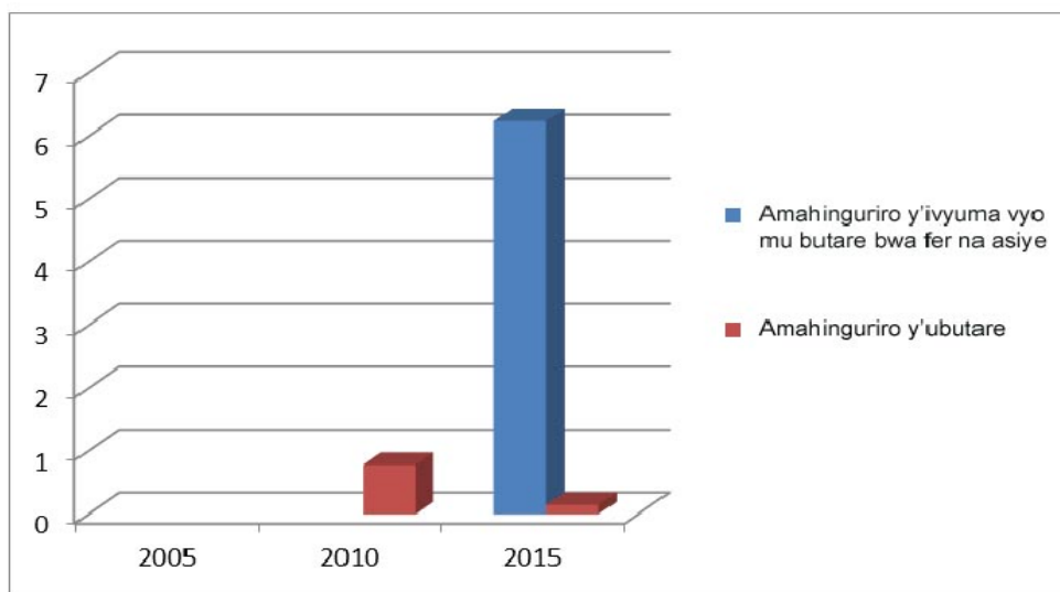
Igicapo ca 10 : Imyitwarire y'irungikwa ry'ivyuka vy'ubumara y'igisata c'ikora ry'amahinguriro n'ikoreshwa ry'ivyahingwe
